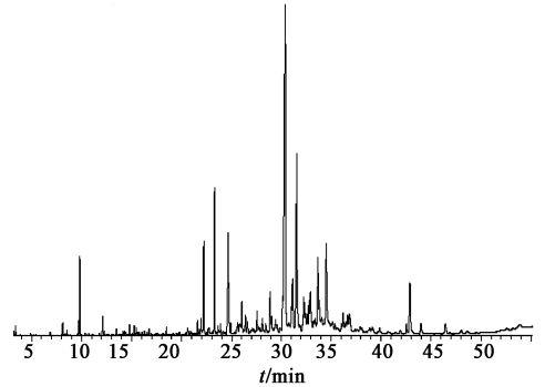
图 1 三脉紫菀挥发油成分总离子流
